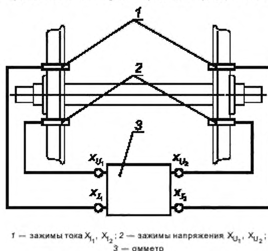
Рисунок 1 — Четырехзажимная схема измерения электрического сопротивления колесной пары
