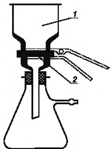
1 — фильтрующая воронка; 2 — опора для фильтра
