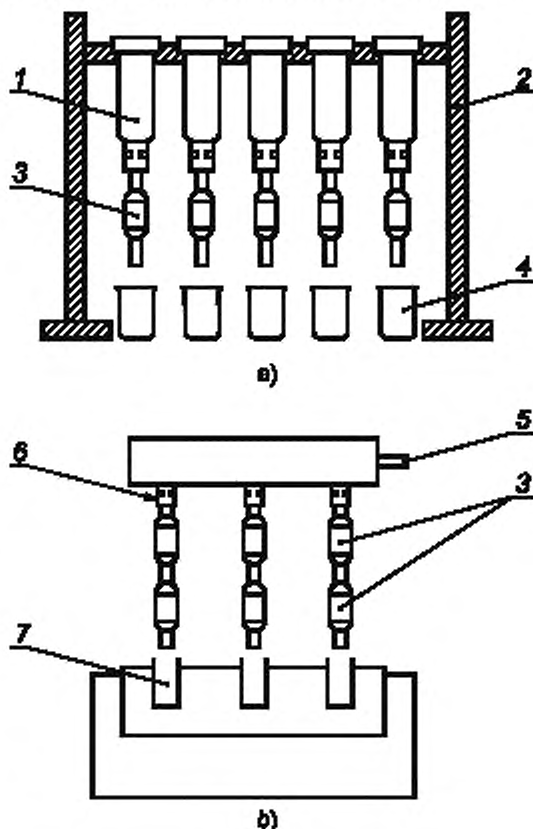
а — устройство для нанесения ДНФГ; б — устройство для сушки картриджей; 1 — стеклянный шприц емкостью 10 мл; 2 — стойка для шприцев; 3 — картриджи; 4 — сливной стакан; 5 — поток N_2 ; 6 — штучер для шприцев; 7 — стаканчик для отходов
