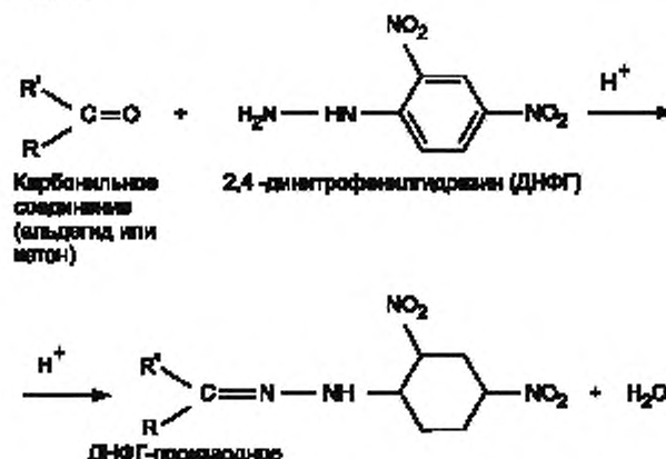
Рисунок 1 — Схема реакции карбонильных соединений с ДНФГ
