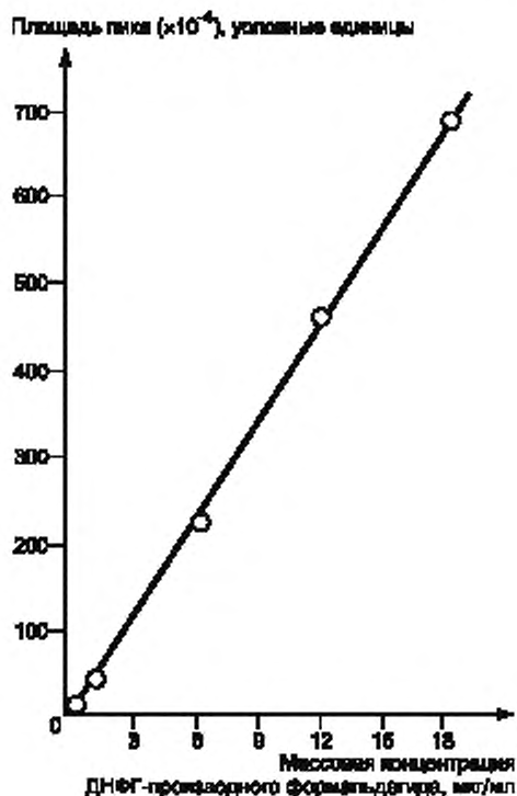
Рисунок 6 — Пример градуировочного графика для формальдегида
