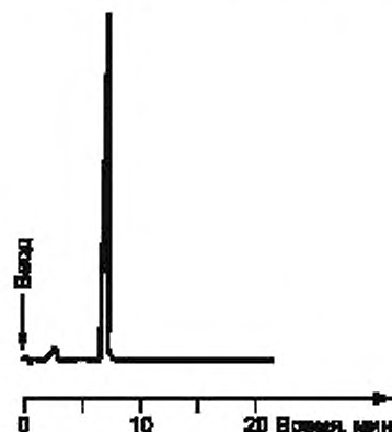
Рисунок 4 — Пример хроматограммы ДНФГ-производного формальдегида
