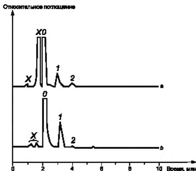
Рисунок 2 — Примеры хроматограмм для формальдегида в потоке воздуха с озоном и без озона
