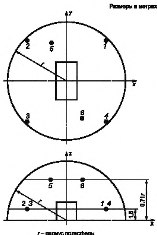
Рисунок 1 — Положения микрофонов на полусфере (см. таблицу 2)
