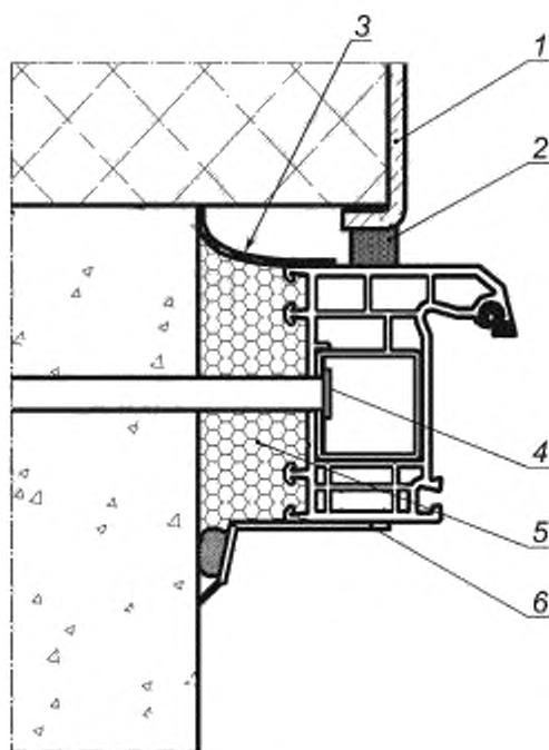
1 — элемент отделки наружного оконного откоса 2 — изоляционная саморасширяющаяся паропроницаемая лента (ПСУЛ); 3 — водоизоляционная паропроницаемая лента; 4 — рамный дюбель; 5 — пенный утеплитель; 6 — нащельник из ПВХ в комбинации с пароизоляционным вкладышем
