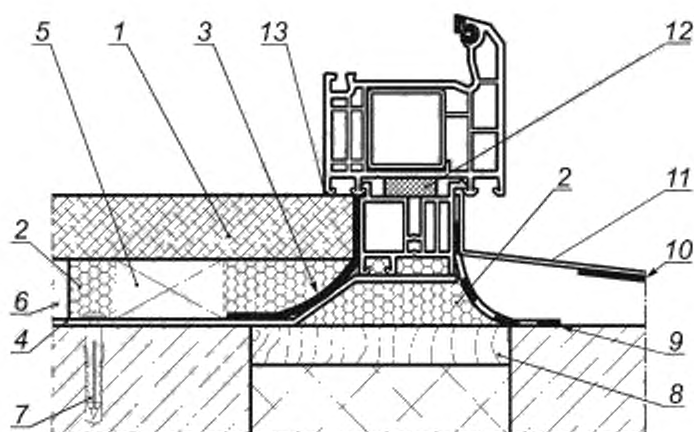
1 — подоконная доска; 2 — пенный утеплитель; 3 — пароизоляционная лента; 4 — гибкая анкерная пластина; 5 — опорная колодка под подоконную доску; 6 — штукатурный раствор; 7 — дюбель со стопорным шурупом; 8 — вкладыш из антисептированного пиломатериала или выравнивающий слой из штукатурного раствора (рекомендуется только для нижнего узла); 9 — водоизоляционная паропроницаемая лента; 10 — шумопоглощающая прокладка; 11 — слив; 12 — изоляционная саморасширяющаяся паропроницаемая лента (ПСУЛ); 13 — тонкий слой герметика
