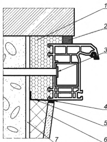
1 — пенный утеплитель; 2 — изоляционная саморасширяющаяся паропроницаемая лента (ПСУЛ); 3 — рамный дюбель; 4 — герметик; 5 — пароизоляционная лента; 6 — панель отделки внутреннего откоса; 7 — штукатурный выравнивающий слой внутреннего откоса
