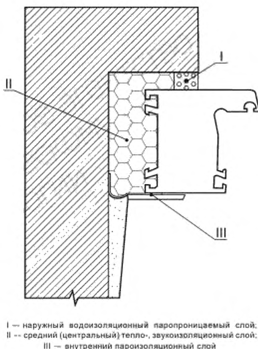
Рисунок 1 — Принципиальная схема монтажного шва
