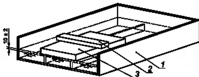
1 — емкость с крышкой; 2 — пригруз, удерживающий образец в частично погруженном положении; 3 — образец
