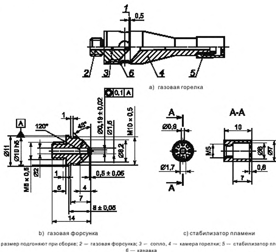
Рисунок 2 — Газовая горелка, лист 1
