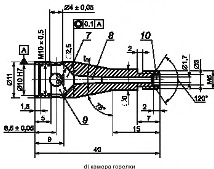
Рисунок 2 — Газовая горелка, лист 1
