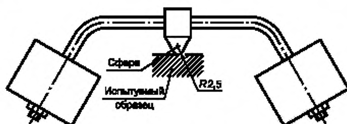
Рисунок 1 — Установка для испытания на теплостойкость
