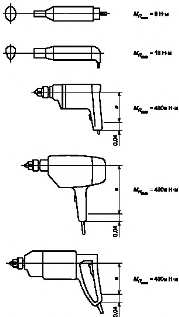
Рисунок 101 — Машины, удерживаемые одной рукой
