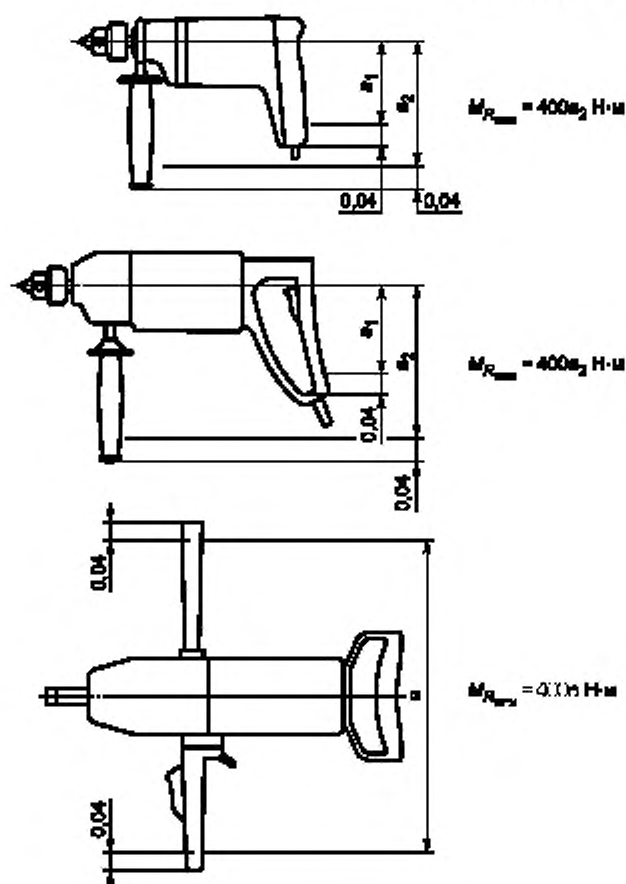
Рисунок 102 — Машины, удерживаемые двумя руками
