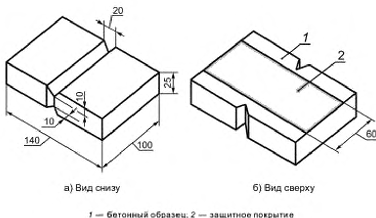
Рисунок 7 — Общий вид образца для определения трещиностойкости
