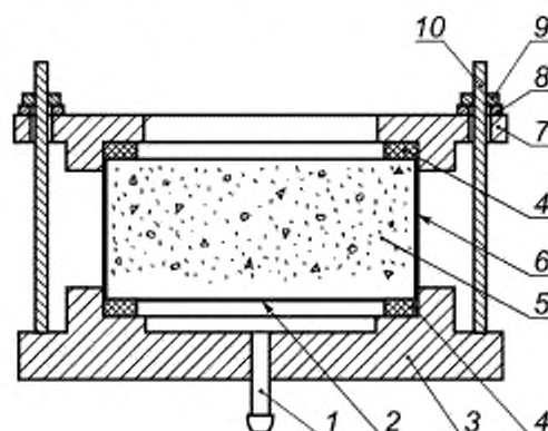
1 — штуцер для подачи воды; 2 — защитное покрытие; 3 — неподвижное гнездо для установки образца; 4 — уплотнительные резиновые кольца; 5 — испытуемый образец; 6 — герметизирующая обмазка или прокладка; 7 — съемная верхняя обойма; 8 — шайба; 9 — гайка; 10 — анкерный стержень с резьбой
