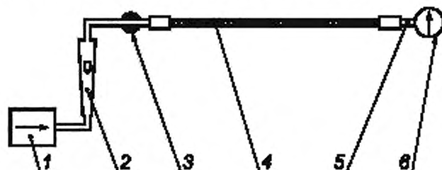
1 — регулируемый источник сжатого газа; 2 — ротамер; 3 — кран; 4 — проверяемый шланг; 5 — переходник к манометру; 6 — манометр
