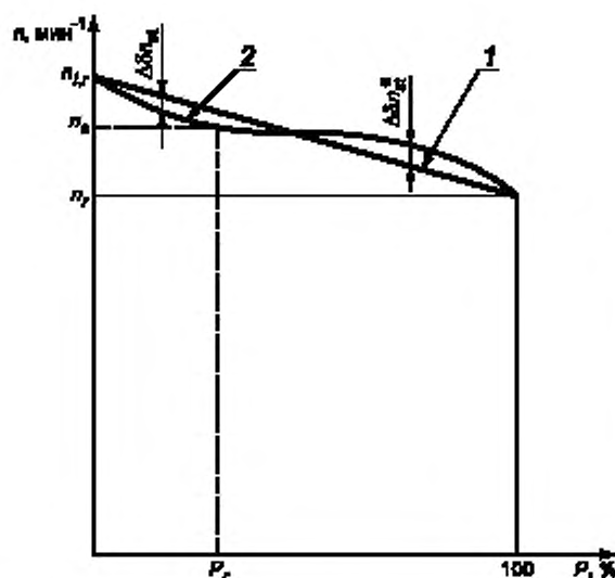
Рисунок 1 — Диапазон уставки частоты вращения
