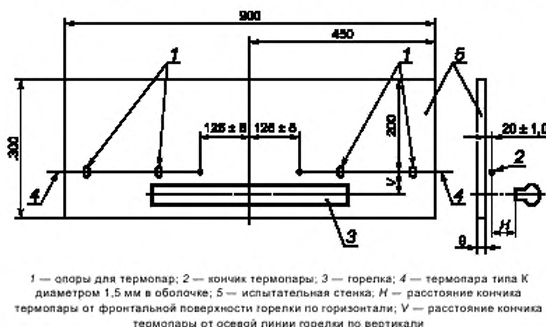
Рисунок А.1 — Расположение системы измерения температуры
