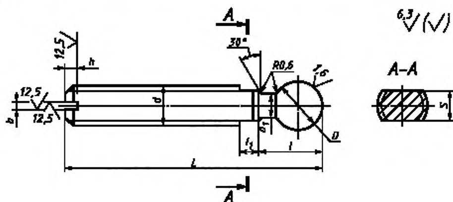
Размеры, мм
