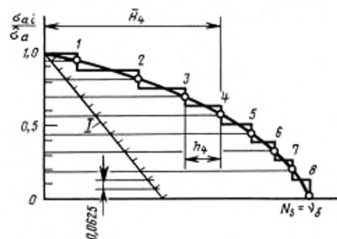
Линейное разбиение спектра нагружения на 8 ступеней
