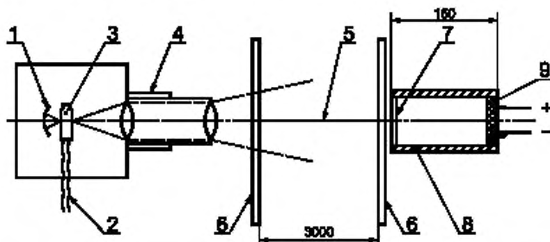
1 — рефлектор; 2 — подача стабилизированного напряжения (12,0 \pm 0,1) \text{ В} (с предельными отклонениями при стабилизации \pm 0,01 \text{ В} ); 3 — галогеновая лампа с кварцевой колбой; 4 — система линз; 5 — световой поток; 6 — окна камеры; 7 — пылезащитное стекло; 8 — трубка с внутренней матовой поверхностью; 9 — фотозлемент
