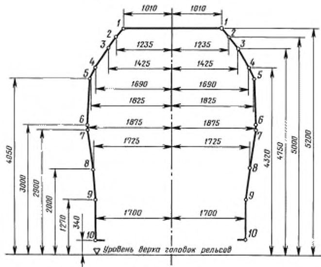
Черт. 8
