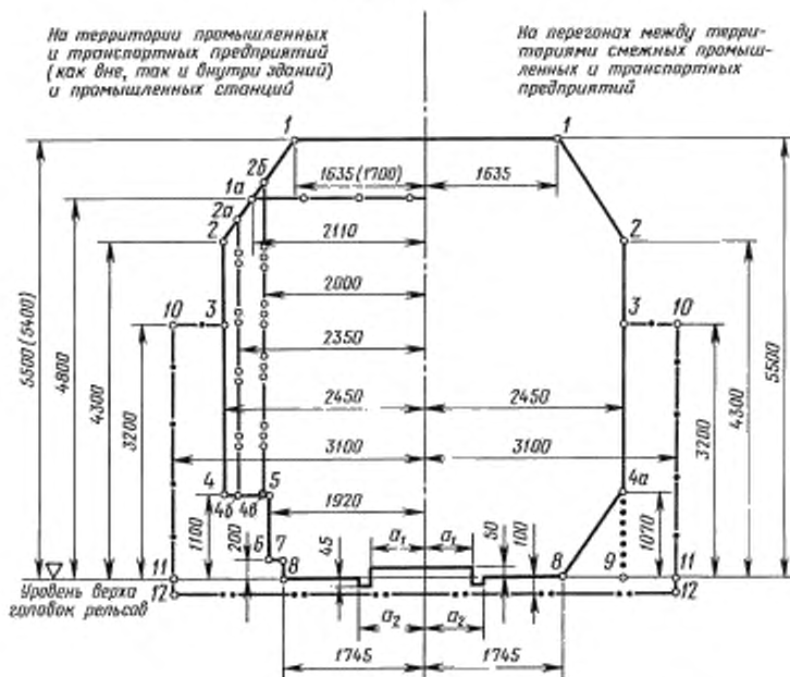
Габарит Сп
