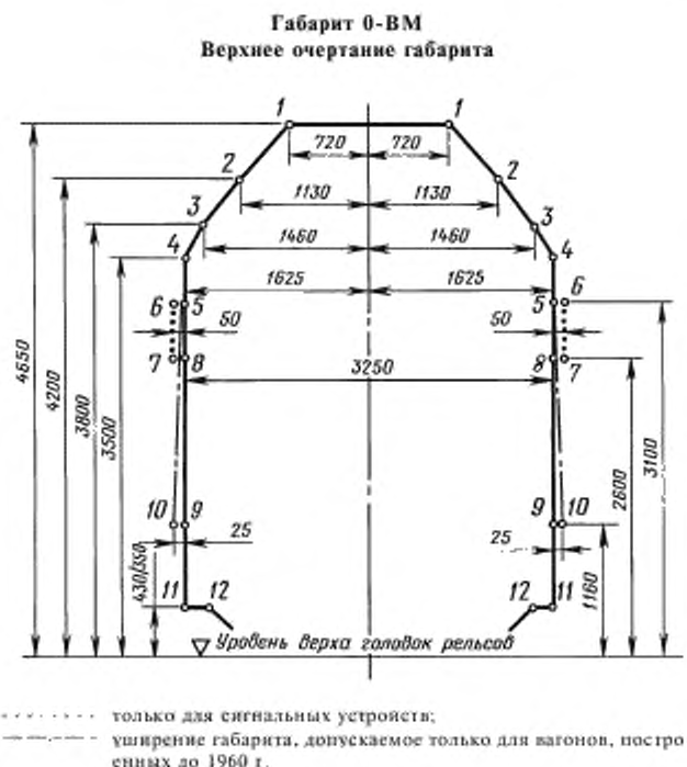
Черт. 13
