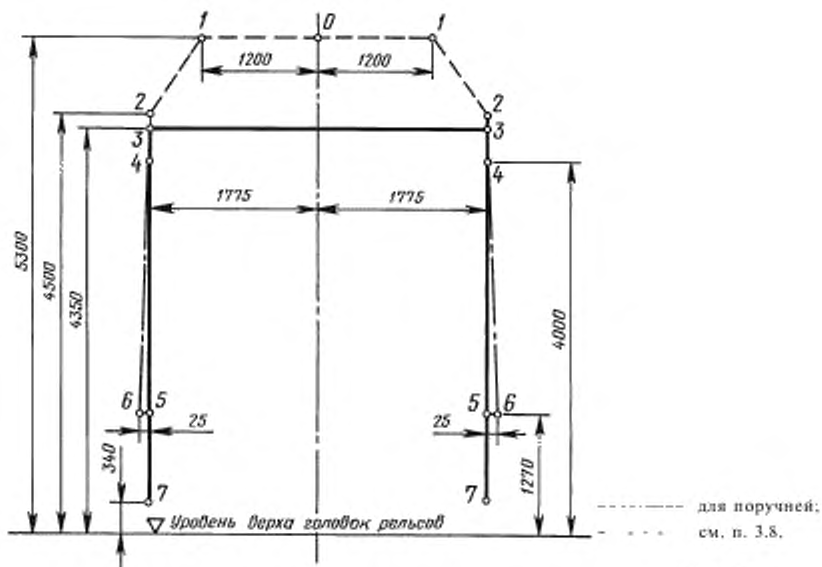
Черт. 9
