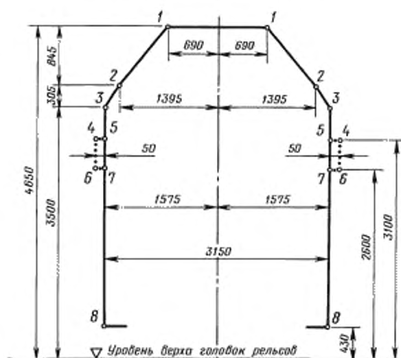
Габарит 02-ВМ Верхнее очертание габарита
