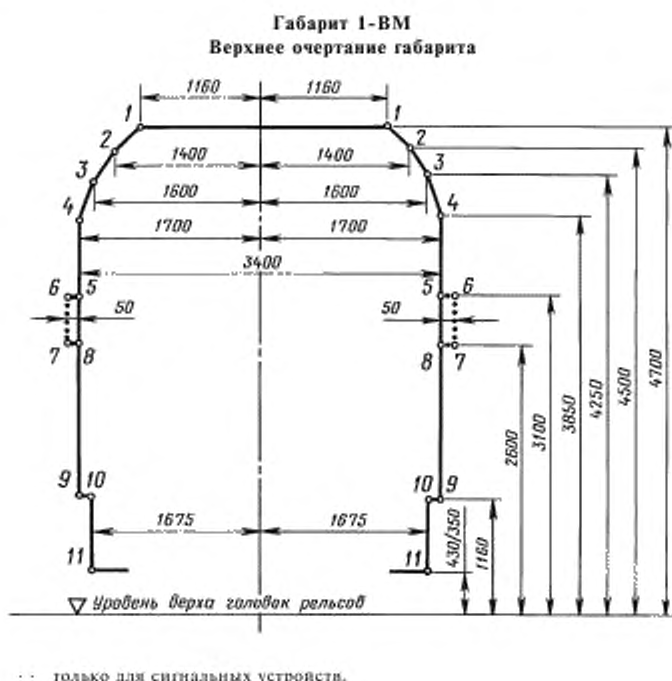
Черт. 12
