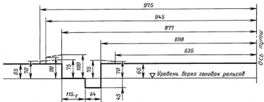
Черт. 5
