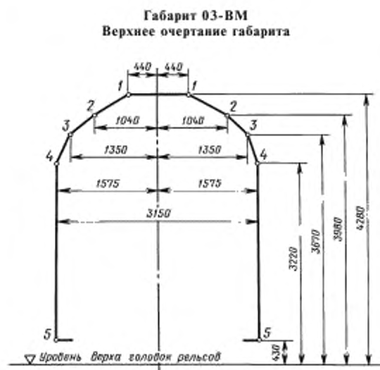
Черт. 16
