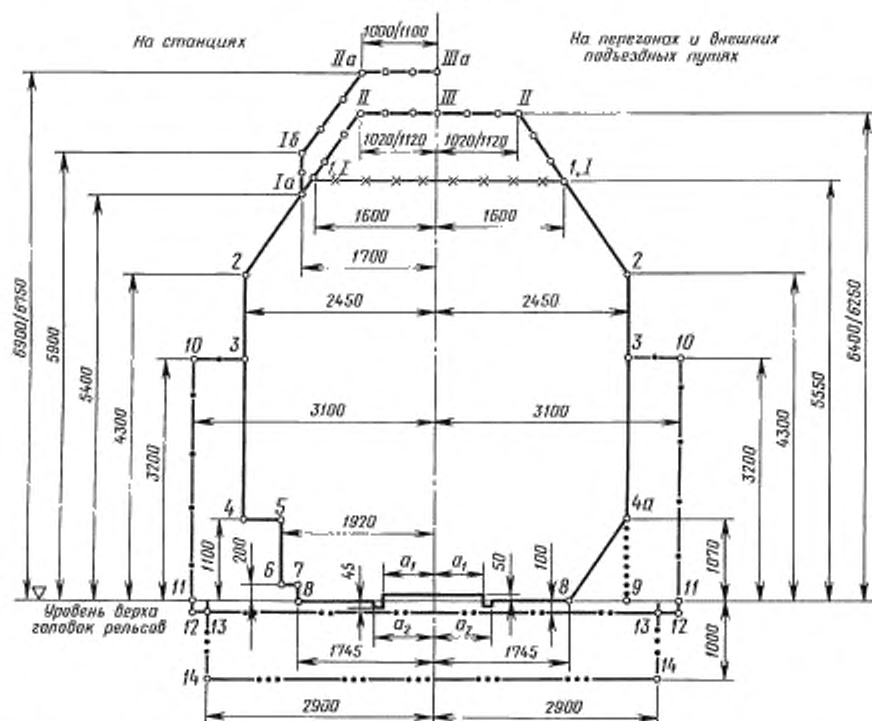
Габарит С
