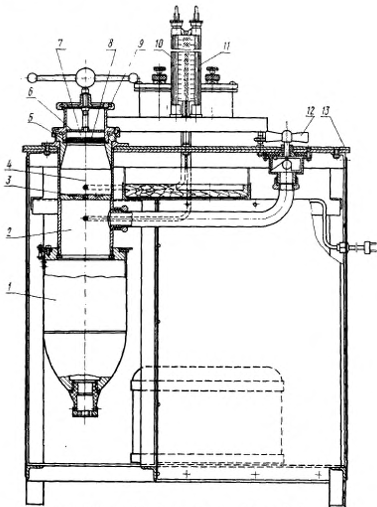
1—вентиль; 2—камера; 3—диафрагма; 4—камера; 5—дно рабочей камеры; 6—крышка рабочей камеры; 7—рабочая камера; 8—фильтр; 9—запорное приспособление; 10—левый манометр; 11—правый манометр; 12—дроссель; 13—стол.
