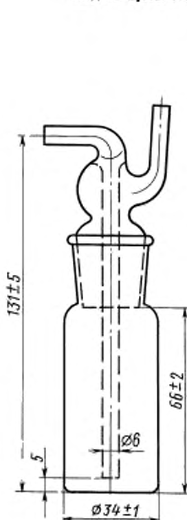
Индикаторная склянка
