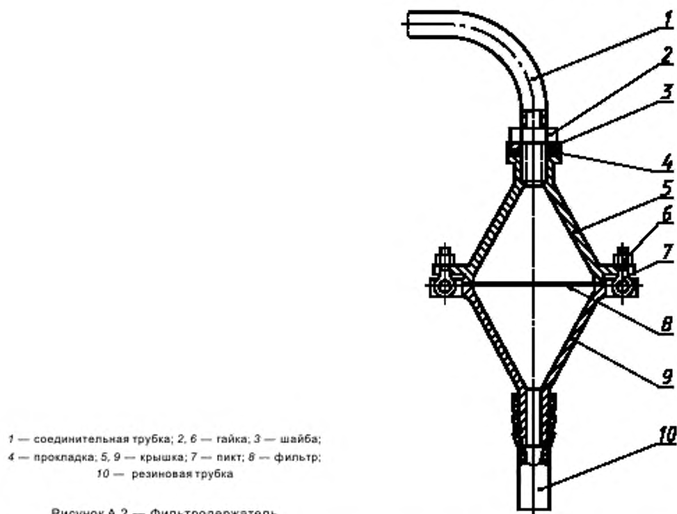
Рисунок А.2 — Фильтродержатель
