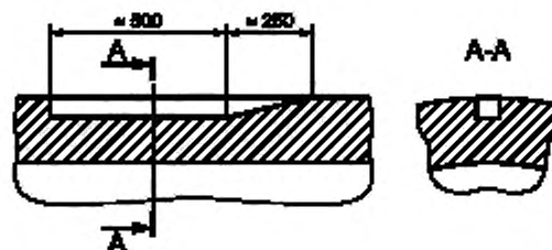
Рисунок 6 — Канавка, обрабатываемая на наружной поверхности трубы
