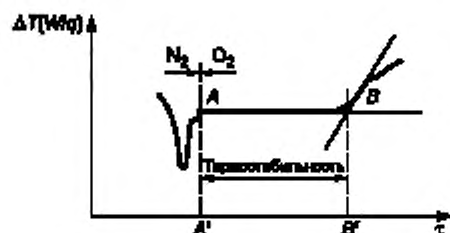
Рисунок 1 — Типичная кривая окислительной термостабильности полиэтилена
