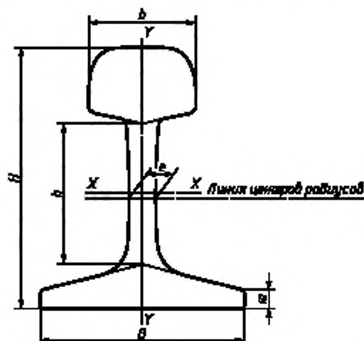
Рисунок 1 — Основные размеры поперечного сечения рельса
