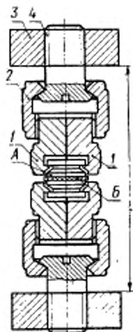
А — металлические диски; Б — резина; 1 — зажим; 2 — гайка; 3 — шайба; 4 — винт
