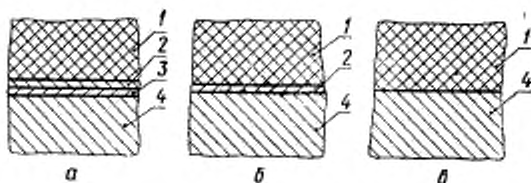
а — при применении двух клеев (методы А и В); б — при применении одного клея; в — при бесклеевом крепление (методы А и В). 1 — резина; 2 — клей; 3 — праймер; 4 — металл
