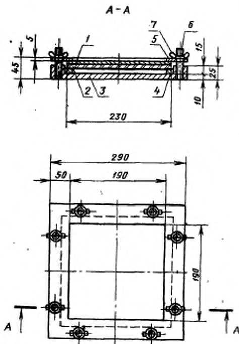
1—образец; 2—плита древесностружечная; 3—основание металлическое; 4—нижняя рамка; 5—рамка прижимная стальная; 6—болт стальной; 7—тайха-барашек
