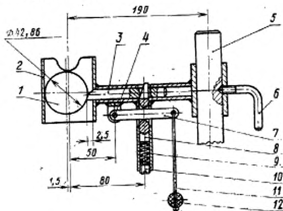
1—шарик; 2—кронштейн; 3—плунжер; 4—ось; 5—штамп; 6—фиксатор; 7—коромысло; 8—илин; 9—пружина; 10—пробка; 11—тросик; 12—рукоятка
