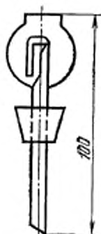
Затвор Геккеля
