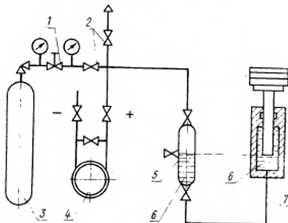
Схема подключения грузопоршневого манометра и разделительного сосуда к поверяемому преобразователю
