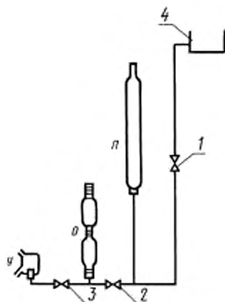
П — поверяемая пипетка; О — образцовая пипетка; У — уравнивающая трубка; 1, 2, 3 — краны; 4 — резервуар для воды
