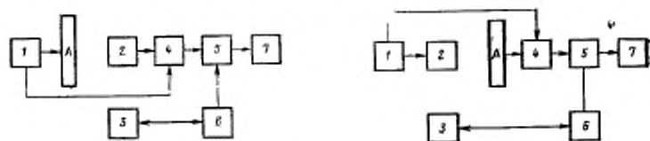
а. Испытуемая антенна в передающем режиме
