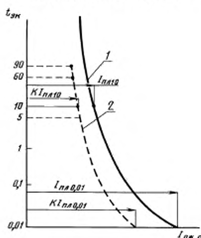
1 — время-токовая характеристика плавления; 2 — время-токовая характеристика предельно допустимых перегрузок I_{пл 10} , I_{пл 0,01} — токи плавления при эквивалентном времени 10 и 0,01 с соответственно
