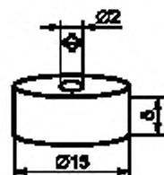
Рисунок 3 — Резиновый наконечник к медицинскому шприцу
