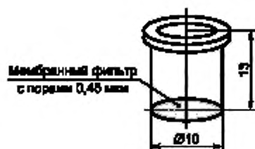
Рисунок 1 — Люминиметрическая полистирольная кювета
