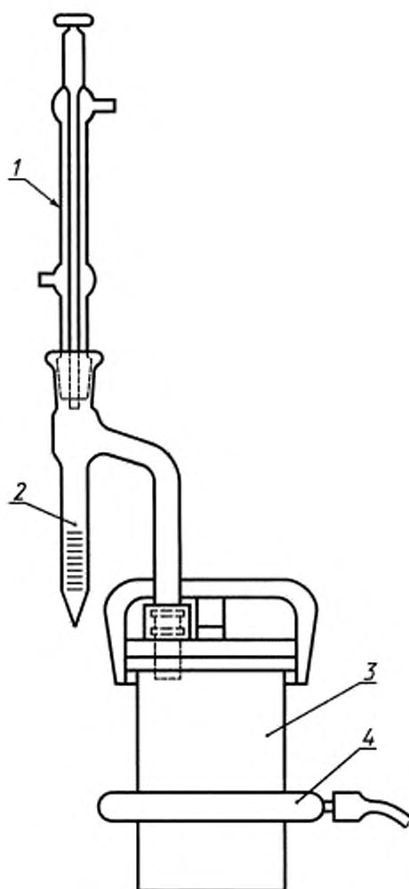
1 — холодильник водный; 2 — приемник-ловушка; 3 — сосуд дистиляционный; 4 — горелка газовая
