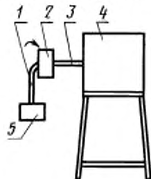
1 — испытуемый образец, 2 — сменный зажим; 3 — вал; 4 — механизм вращения; 5 — груз
