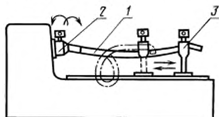
1 — испытуемый образец; 2 — вращающийся зажим; 3 — зажим с возвратно-поступательным движением
