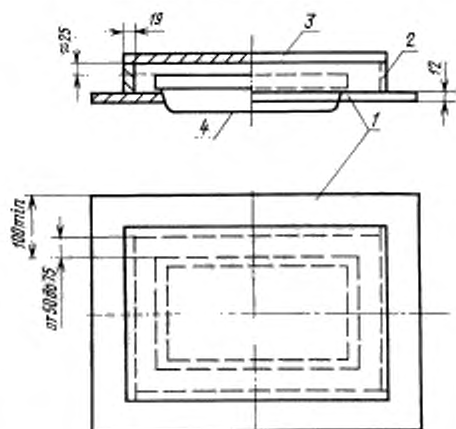
1 — основа, 2 — боковая стенка, 3 — верхняя стенка, 4 — испытуемый светильник
