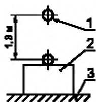
1 — стальной шарик; 2 — светильник; 3 — опорная поверхность Черт. 7а
