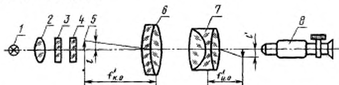
1—источник света; 2—конденсор; 3—молочное (опаловое) стекло; 4—светофильтр; 5—штриховая шкала; 6—объектив коллиматора; 7—испытуемый объектив; 8—микро- скоп с окуляр-микрометром или микрометрическим поперечным перемещением
