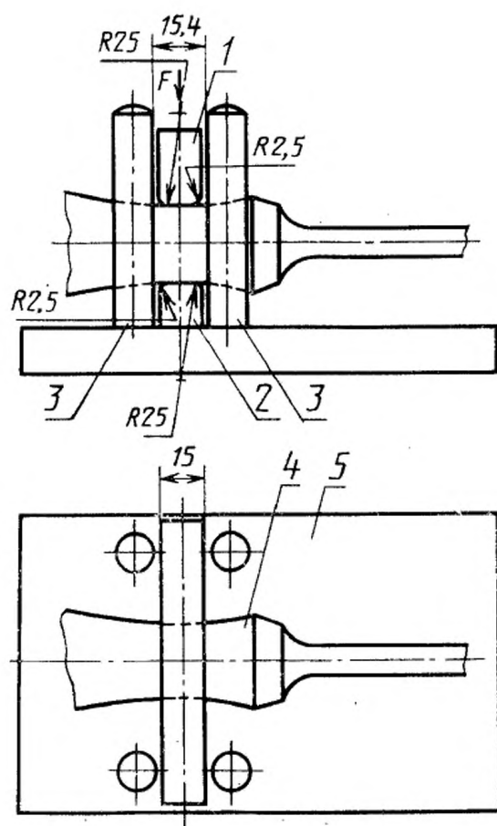
1—верхняя подвижная губка; 2—нижняя губка; 3—направляющие; 4—испытываемый светильник; 5—плита; F —усилие сжатия
