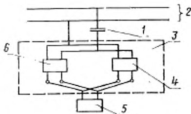
1—разделительный конденсатор; 2—источник постоянного тока; 3—фильтр ДК; 4—фильтр нижних частот Д; 5—электронный вольтметр; 6—фильтр верхних частот К.
