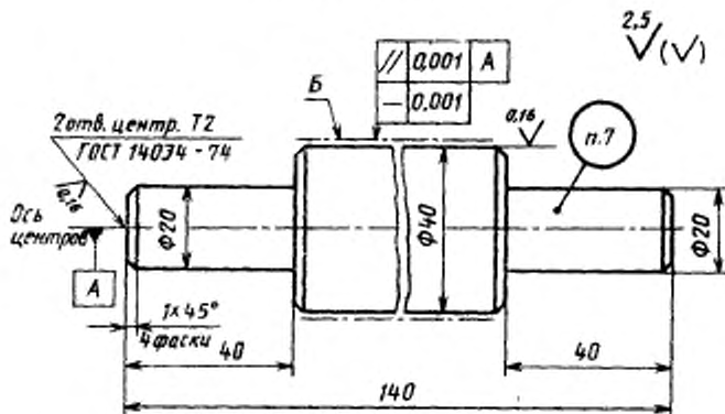
Цилиндрическая оправка
