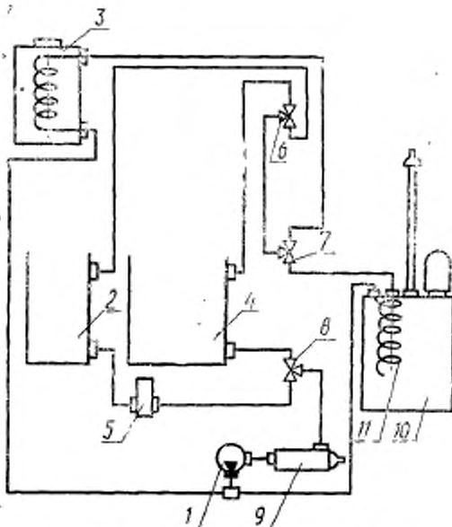
1—насос; 2—бак проточных первичных преобразователей; 3—холодильник; 4—бак погружных первичных преобразователей; 5—проточный первичный преобразователь; 6—8—трекходоосы явры; 9—термометр сопотопления; 10—термостат; 11—элевик
