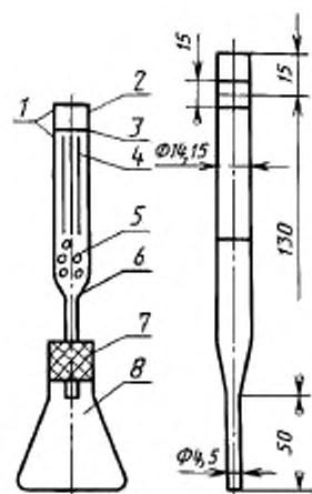
1 — стеклянные крючки; 2 — отрезная часть трубки; 3 — квадрат бромнортутной бумаги; 4 — полоски бумаги; 5 — тампон из ваты; 6 — стеклянная трубка; 7 — резиновая пробка; 8 — коническая колба
