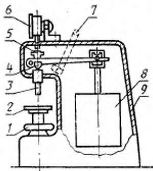
1—гайка-маховик; 2—подъемный столик; 3—индентор; 4—призма рычага основной нагрузки; 5—шпindel с грузом предварительной нагрузки; 6—отсчетное устройство; 7—рукоятка приложения и снятия основной нагрузки; 8—грузы для основной нагрузки; 9—корпус
