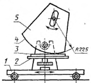
1—площадка; 2—стол; 3—образец; 4—шлифовальная шкурка; 5—рабочий элемент
