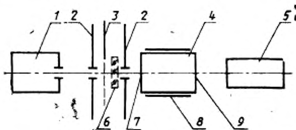
1—источник света; 2—светозащитная диафрагма; 3—заслонка; 4—ЭОП; 5—яркомер; 6—светофильтр; 7—фотокаод; 8—держатель ЭОП; 9—экран
