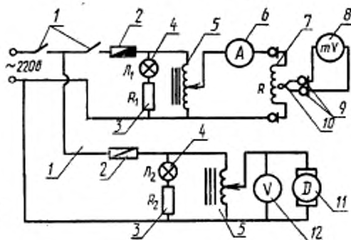
Электросхема центрифуги
