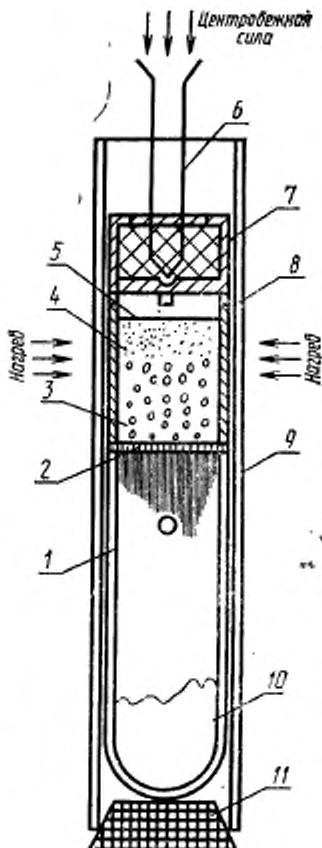
Загрузочный патрон
