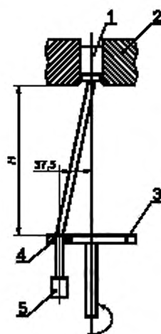
1 — зажим; 2 — подставка; 3 — плата; 4 — втулка; 5 — груз
