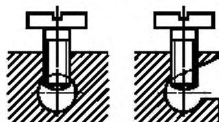
Торцевые зажимы с прямым усилием прижатия жилы проводника без прижимной пластины
