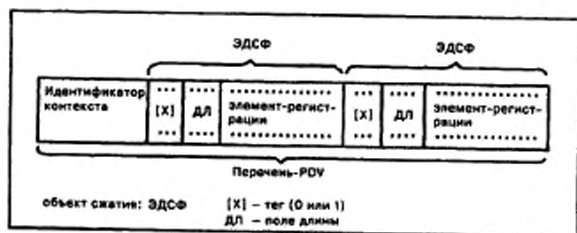
Рисунок 5 — Метод сжатия INTAR-СП
