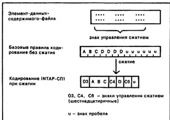
Рисунок 7 — Пример кодирования при использовании INTAP-СП1
