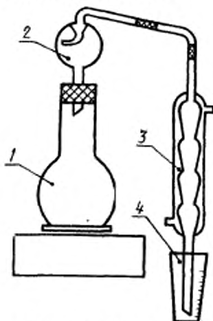
1 — колба; 2 — каплеуловитель; 3 — холодильник; 4 — мензурка
