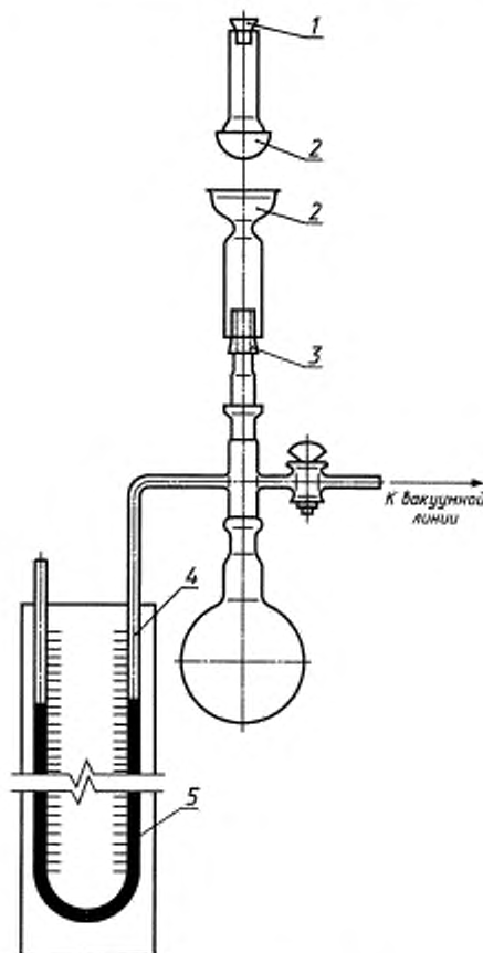
1 — резиновая пробка; 2 — испытуемый шлиф; 3 — резиновая пробка или трубка по размеру испытуемого соединения; 4 — шкала с диапазоном измерения давления приблизительно от 350 до 760 мм рт.ст. (45—100 кПа), с ценой деления 1 мм (0,133 кПа); 5 — ртутная U-образная манометрическая трубка
