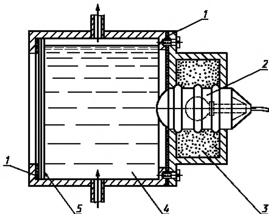
1 — уплотнение; 2 — испытуемый образец; 3 — песок с размером частиц около 1 мм; 4 — вода; 5 — стеклянная перегородка
