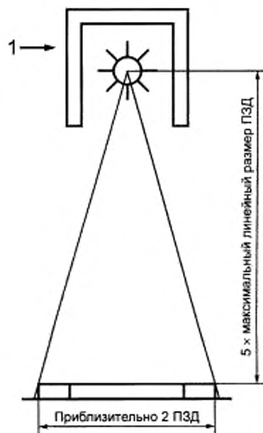
Рисунок 5 — Расположение источника для определения собственных функций (3.2.2, 3.3.1, 3.4 и 3.6)
