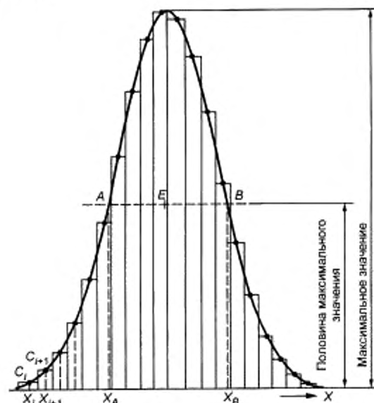
Рисунок 7 — Измерение ПОЛНОЙ ШИРИНЫ НА УРОВНЕ ПОЛОВИНЫ МАКСИМУМА (ПШПМ)
