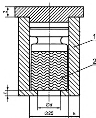
Рисунок 6 — Небольшой жидкий источник с ЗАЩИТОЙ БЛОКА ДЕТЕКТИРОВАНИЯ
