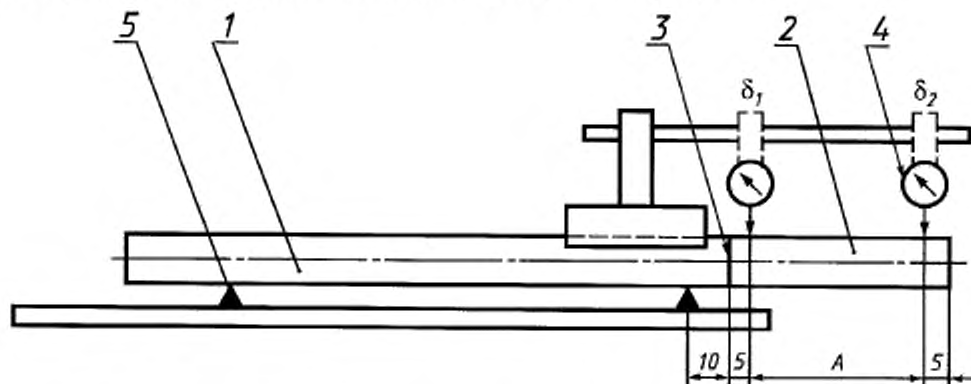
1 — труба; 2 — деталь приварного замка; 3 — сварное соединение (шов); 4 — индикатор часового типа; 5 — ножевая опора; \delta_1, \delta_2 — сечения, в которых измеряют биение; A — расстояние между сечениями
