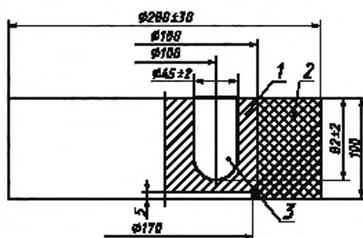
Рисунок Б.1 Алюминиевый блок с шестью гнездами
